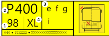
Etiqueta de carga del tren
