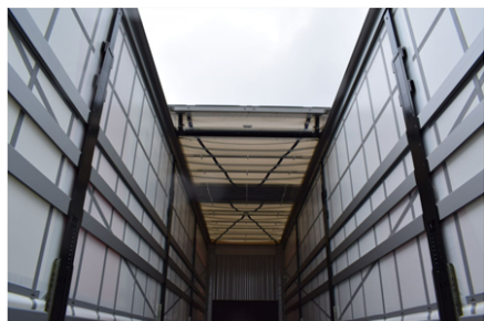
Elevación del techo
