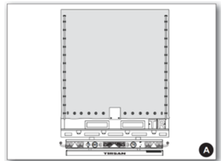
Parte trasera del semirremolque
