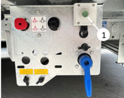
Botón del muelle en la placa del brazo
