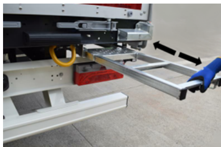
Escalera plegable deslizante
