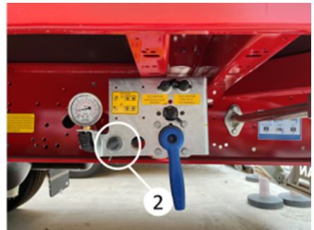
Hohe Fahrhöhe
