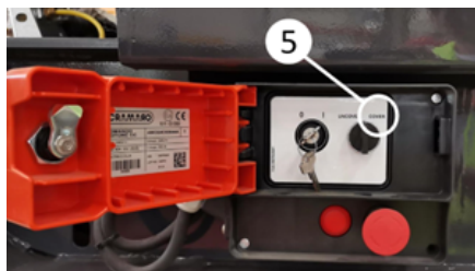
Schließen der Plane mit dem Steuergerät
