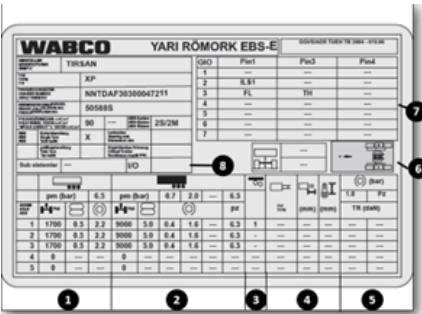
Bremsenaufkleber
