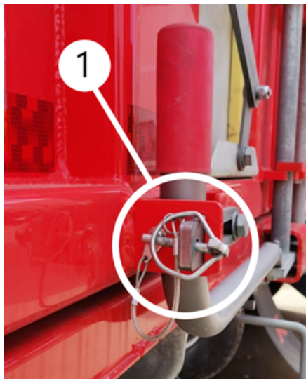
Stift des Türverriegelungshebels
