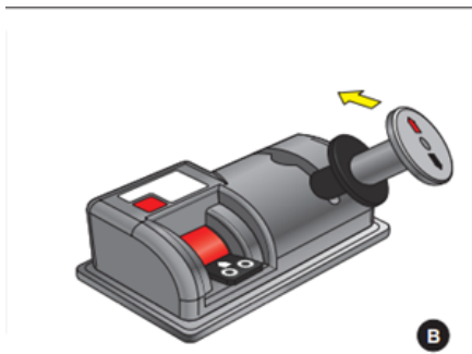
Drücken Sie den Hebel zum Heben und Senken nach vorne in Richtung des roten Pfeils auf dem Hebel.
