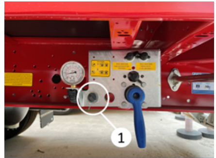
Niedrige Fahrhöhe
