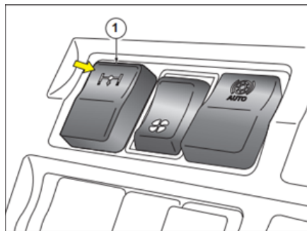
Umschalten des PTO-Schalters in die obere Position
