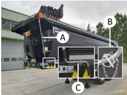
Herausnehmen des Schwenkrohrs aus seiner Aufnahme
