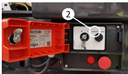
Öffnen der Plane über das Steuergerät
