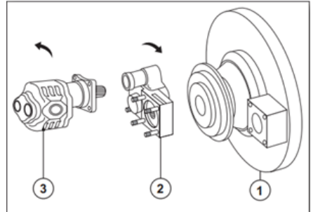
Verbindung Pumpe - PTO
