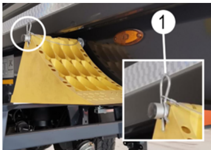
Unterlegkeil
