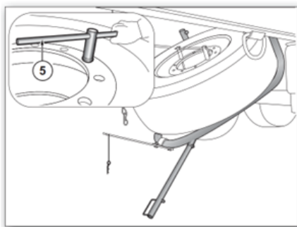
Absenken des Reserve- rads
