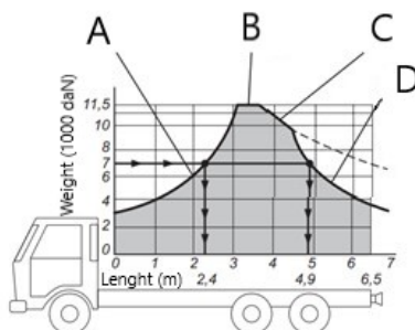
Einwirkende Kräfte
