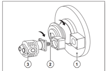
Pumpe - PTO-Anschluss
