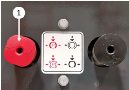
Federbelastete Handbremse
