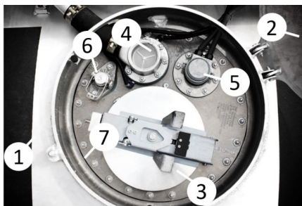
Mannlochbereich
