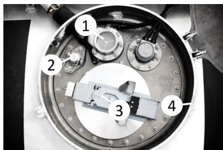
Mannlochbereich
