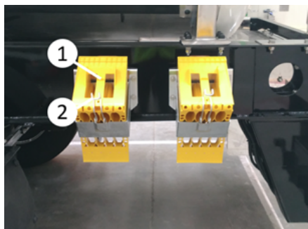
Taschentyp Radkeil
