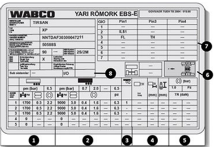
Bremsenaufkleber
