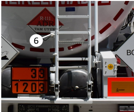
Ventilmechanismus
