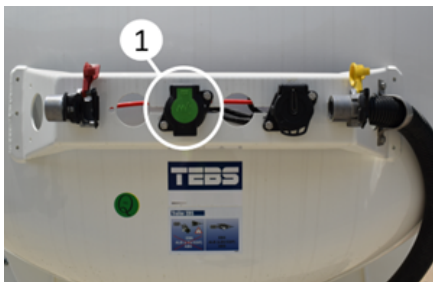
15-polige Buchse
