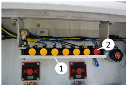
Pneumatischer Steuerblock
