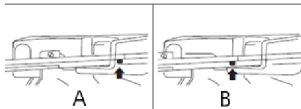
5. Radverriegelungssystem
