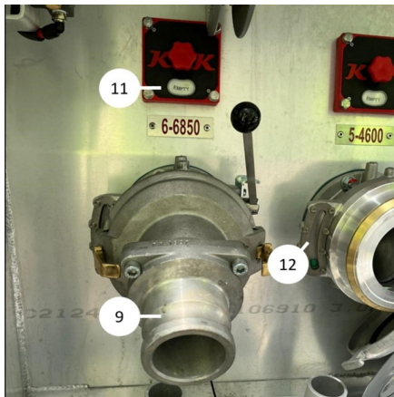
API-Kupplungen
