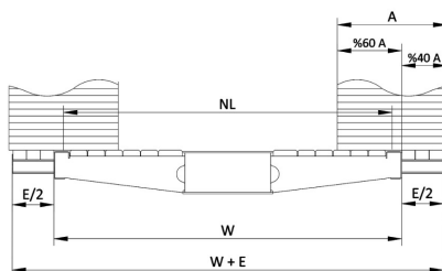
Carga sobre soportes de expansión
