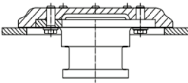
King Pin de 3,5 pulgadas
