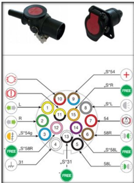
Enchufe ISO12098
