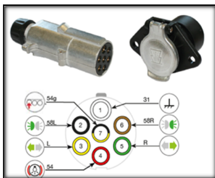
Enchufe ISO1185
