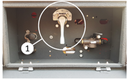
Posición de conducción con suspensión neumática y mando manual
