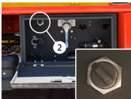
Pneumatyczny trzpień blokujący Przelącznik
