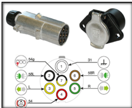
Gniazdo ISO1185
