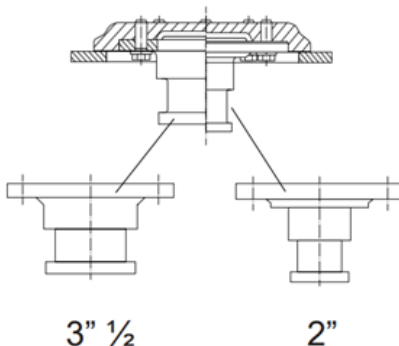
2-calowy sworzeń królewski
