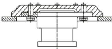
3,5 cala sworzeń królewski
