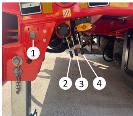
Przycisk obsługi pompy i dźwignie sterowania rampą
