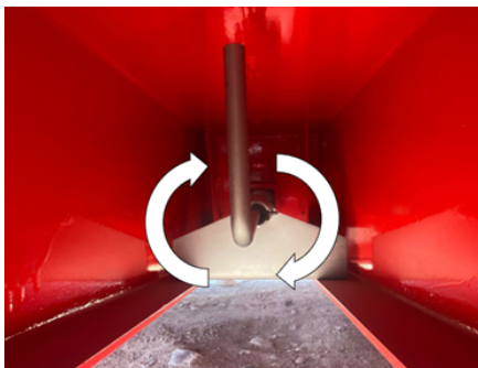
Obrót sworznia zamykającego
