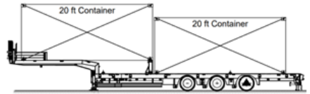
Transport kontenera 2x20 ft z gęsią szyją
