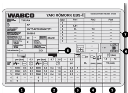
Naklejka do hamulców
