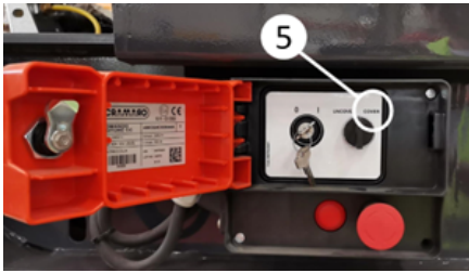
Schließen der Plane mit dem Steuergerät
