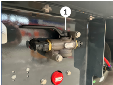
Feststellbare Nachlaufachse
