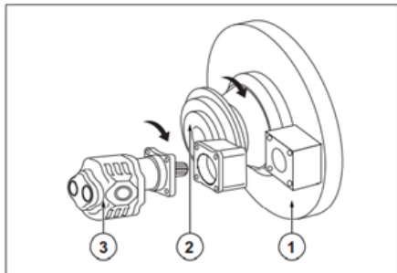
Pumpe - PTO-Anschluss
