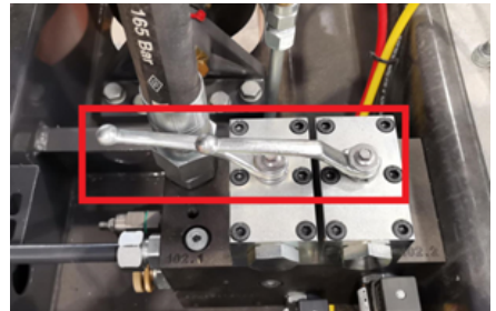
Schalten Sie das Ventil auf die Position "on".
