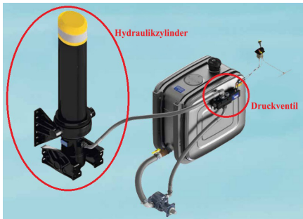
Hydraulikanschluss-Diagramm
