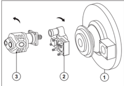
Verbindung Pumpe - PTO
