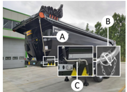
Herausnehmen des Schwenkrohrs aus seiner Aufnahme
