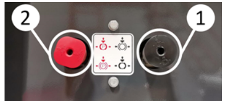
Bedienelemente der Bremse
