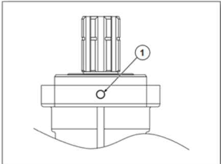
Ölwarnbohrung
