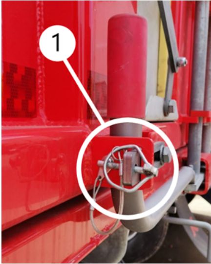
Stift des Türverriegelungshebels
