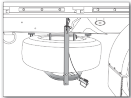
Ersatzradhalter
