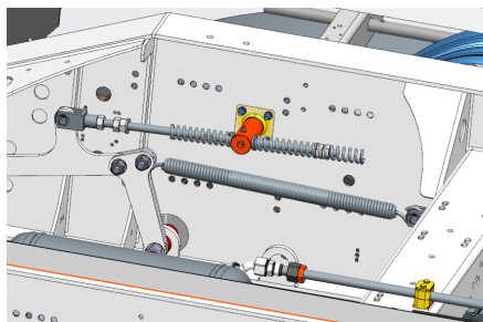
Federmechanismus
