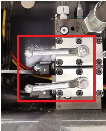
Schalten Sie das Ventil auf die Position "off".
