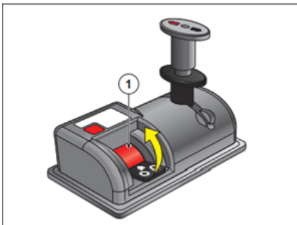
Einschalten der PTO
